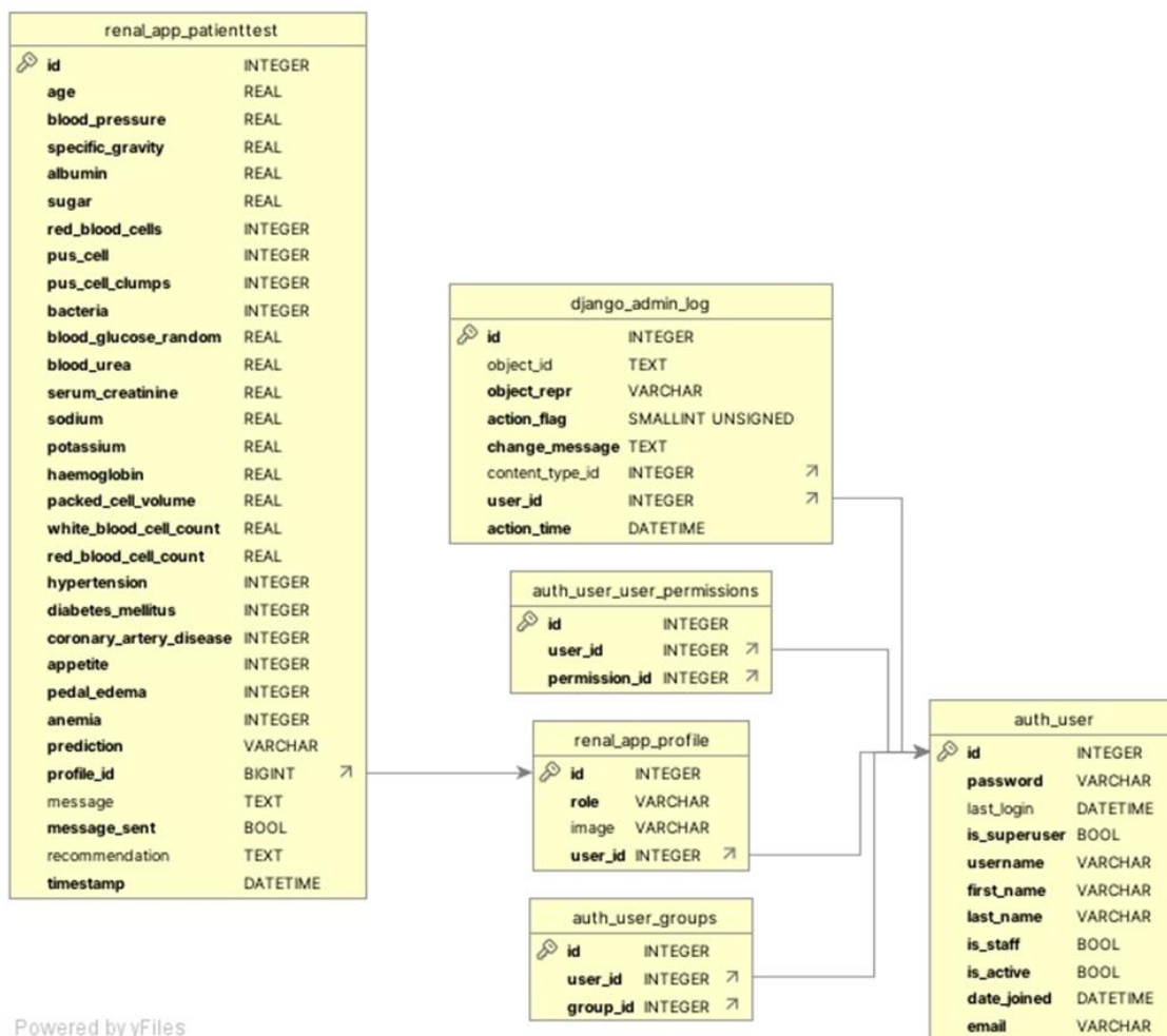
Slika 3.1. Odnosi entiteta
