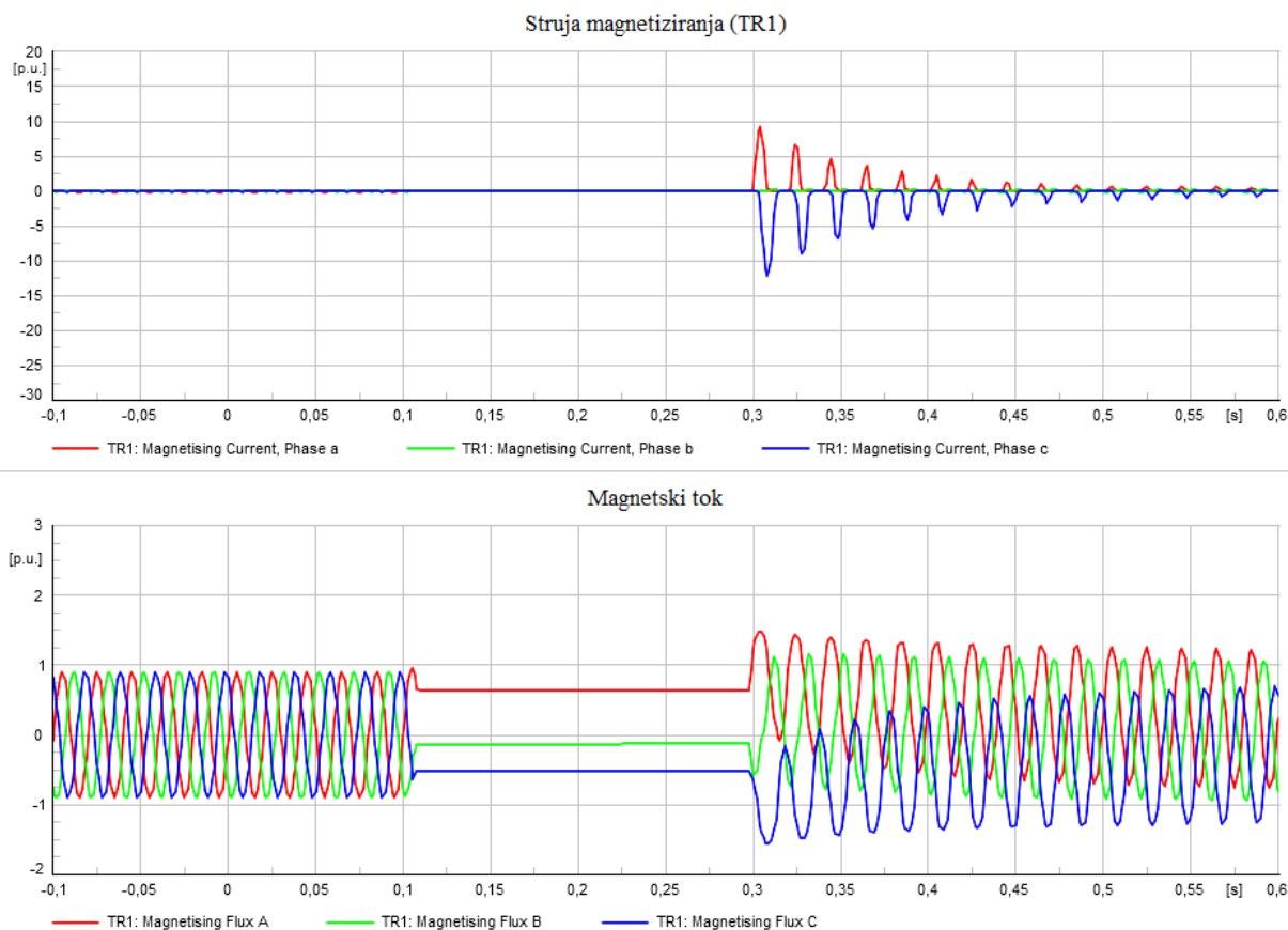
Slika 4.17. Prikaz struja magnetiziranja i magnetskog toka za vrijeme uključenja transformatora
