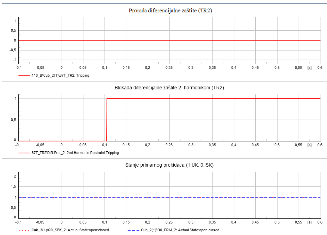
Slika 4.35. Karakteristike diferencijalnog releja na transformatoru 2 (TR2) za vrijeme uključjenja transformatora TR1
