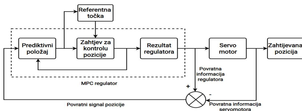
Slika 4.3. Blok dijagram MPC regulatora servomotora [31]
