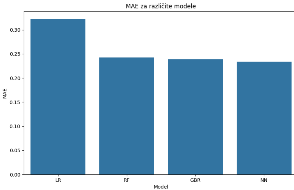
Slika 5.34. Usporedba MAE.
