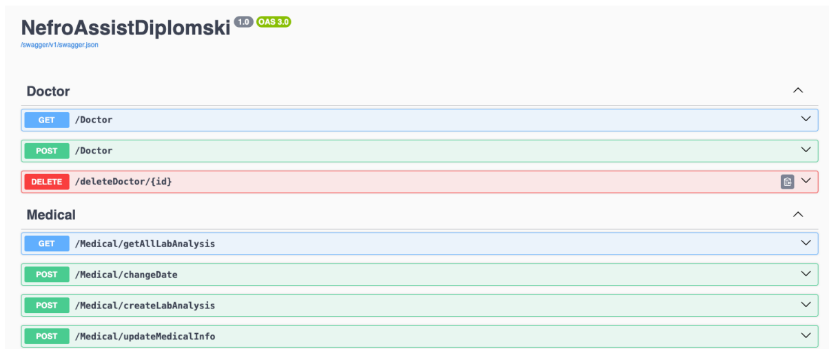
Slika 4.13. Prikaz sučelja alata swagger
