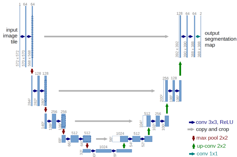
Slika 2.2. U-Net arhitektura [2]
