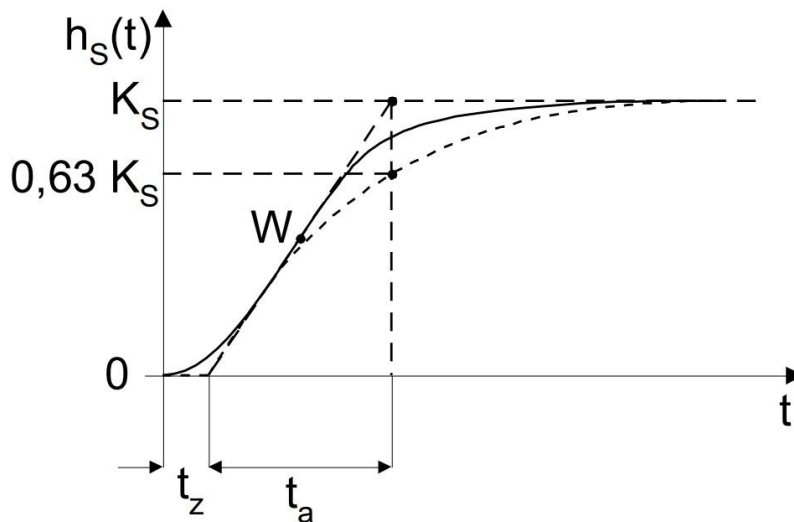
Sl 3.5. Prijelazna funkcija procesa
