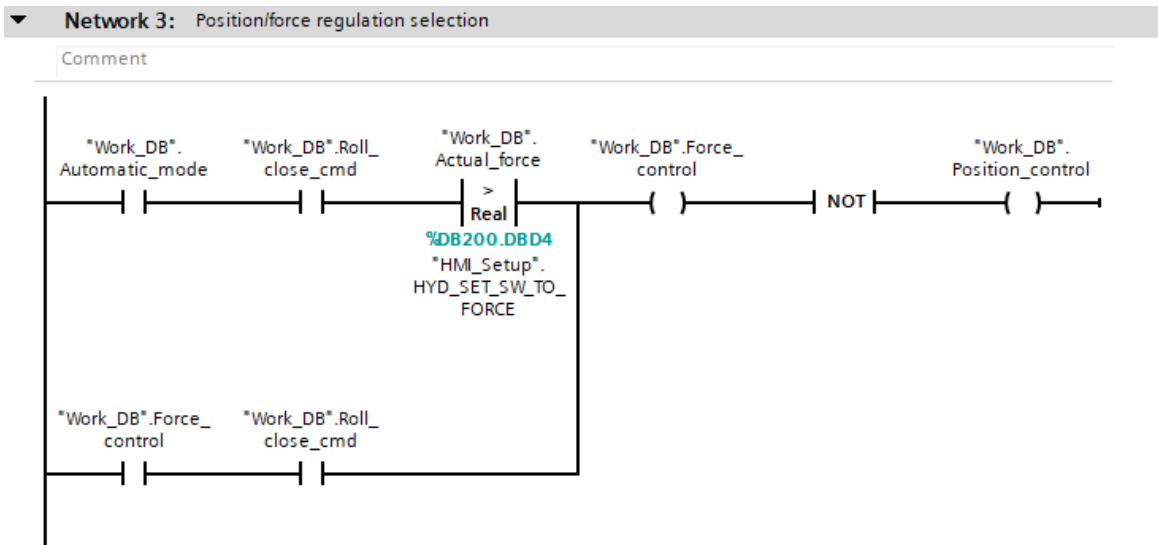
Sl. 4.27. Odabir regulacije pozicije i pritiska
