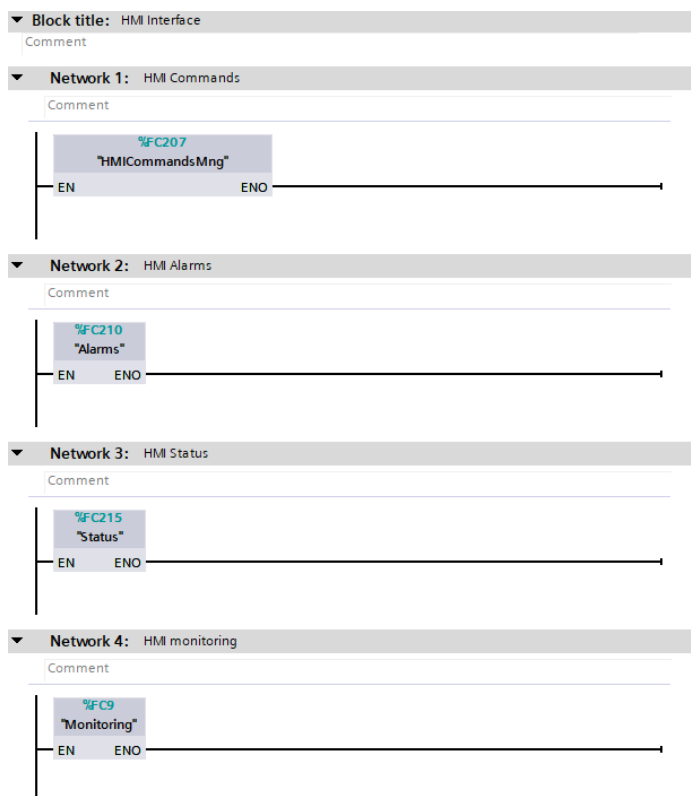
Sl. 4.10. Funkcija HMI_Interface
