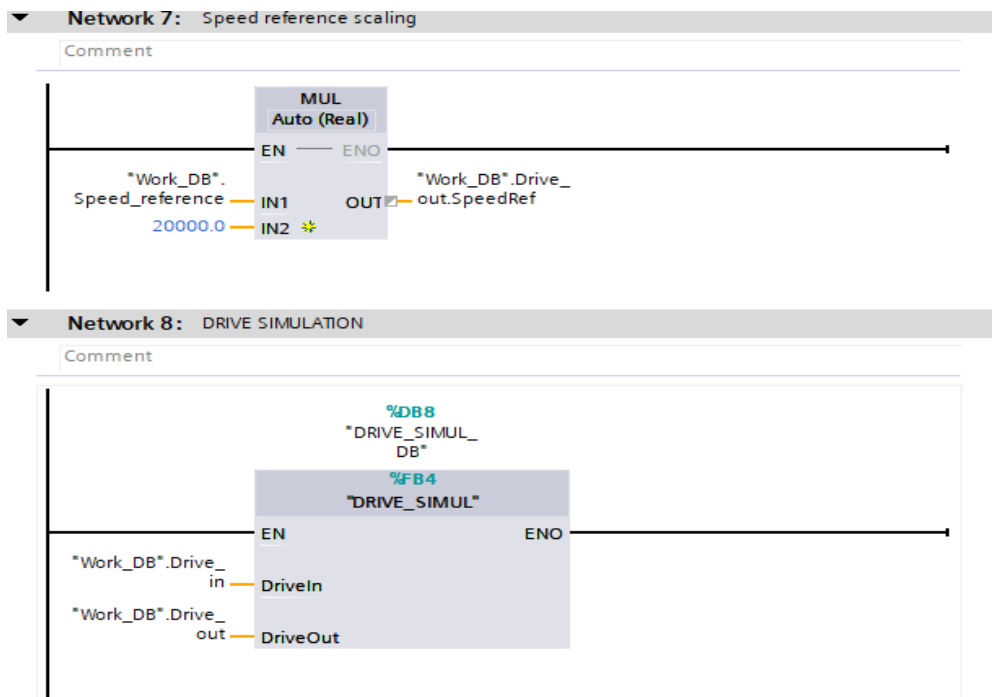
Sl. 4.28. Skaliranje i predaja reference pogonu
