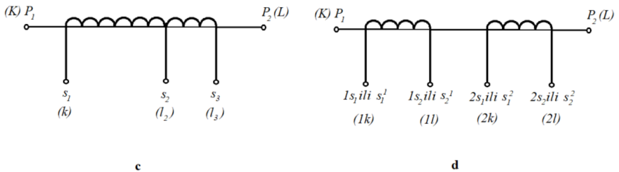
Slika [2.21]. c-strujni mjerni transformator s dvije ili više jezgara i namotom s odvojcima na sekundarnoj strani, d - strujni mjerni transformator s dvije ili više jezgara, gdje priključci sekundarnog namota nose broj pripadne jezgre [29]
