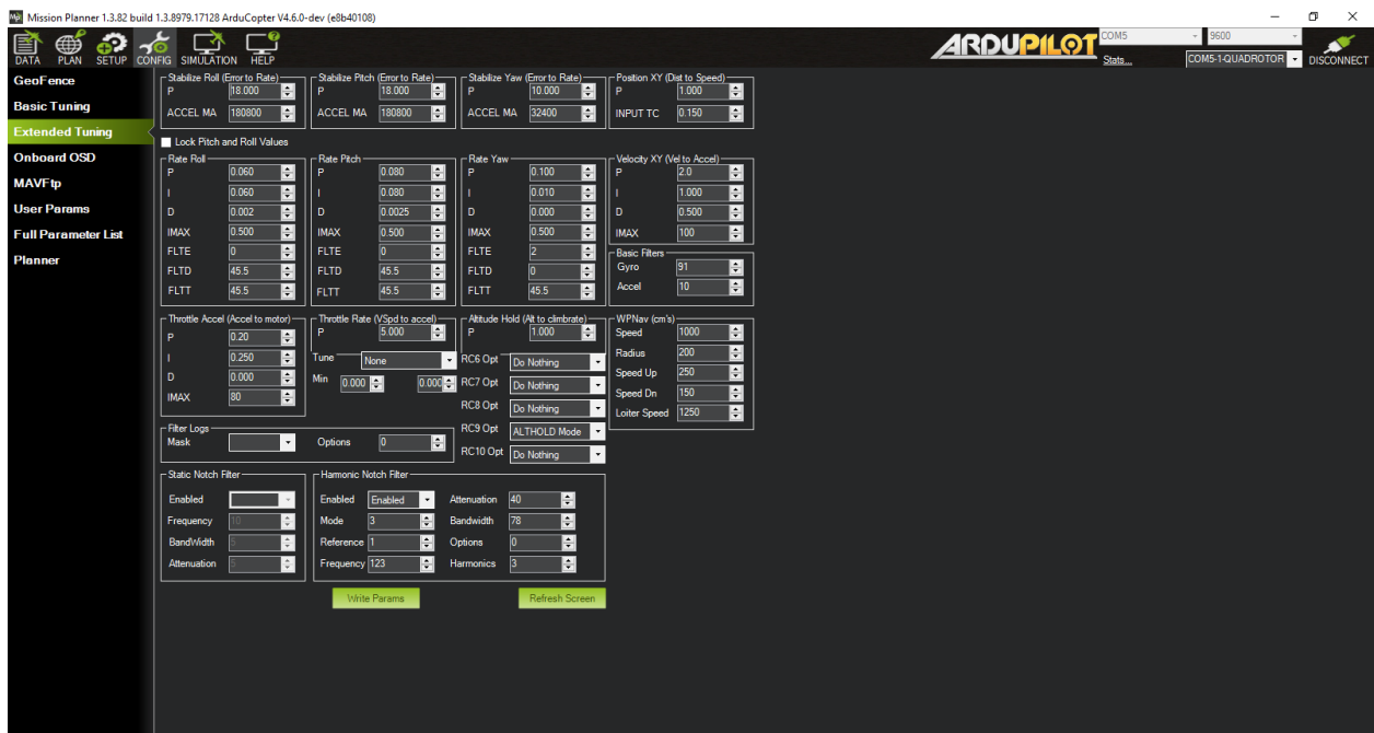
Slika 5.6. Prikaz parametara za PID regulator u Mission Planner-u
