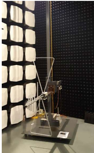
Slika 6.6. Prikaz položaja antene kod određivanja referentne razine izračenog električnog polja
