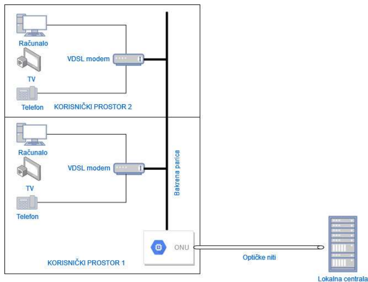
Slika 3.4. Arhitektura FTTB sustava [13]
