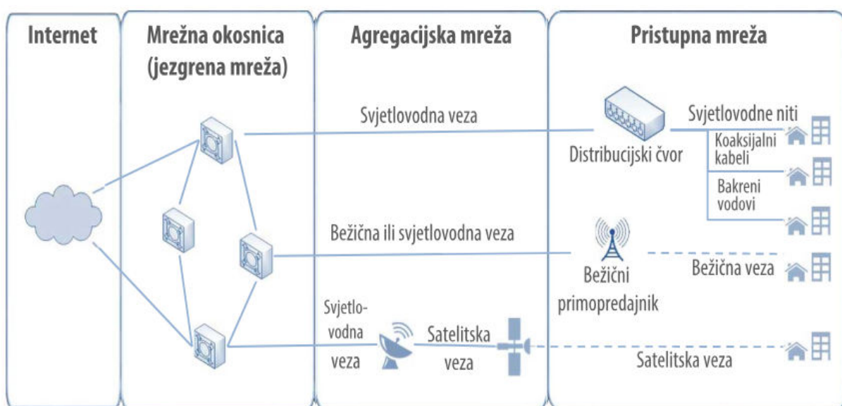
Slika 2.1: Struktura širokopojasne mreže [1]
