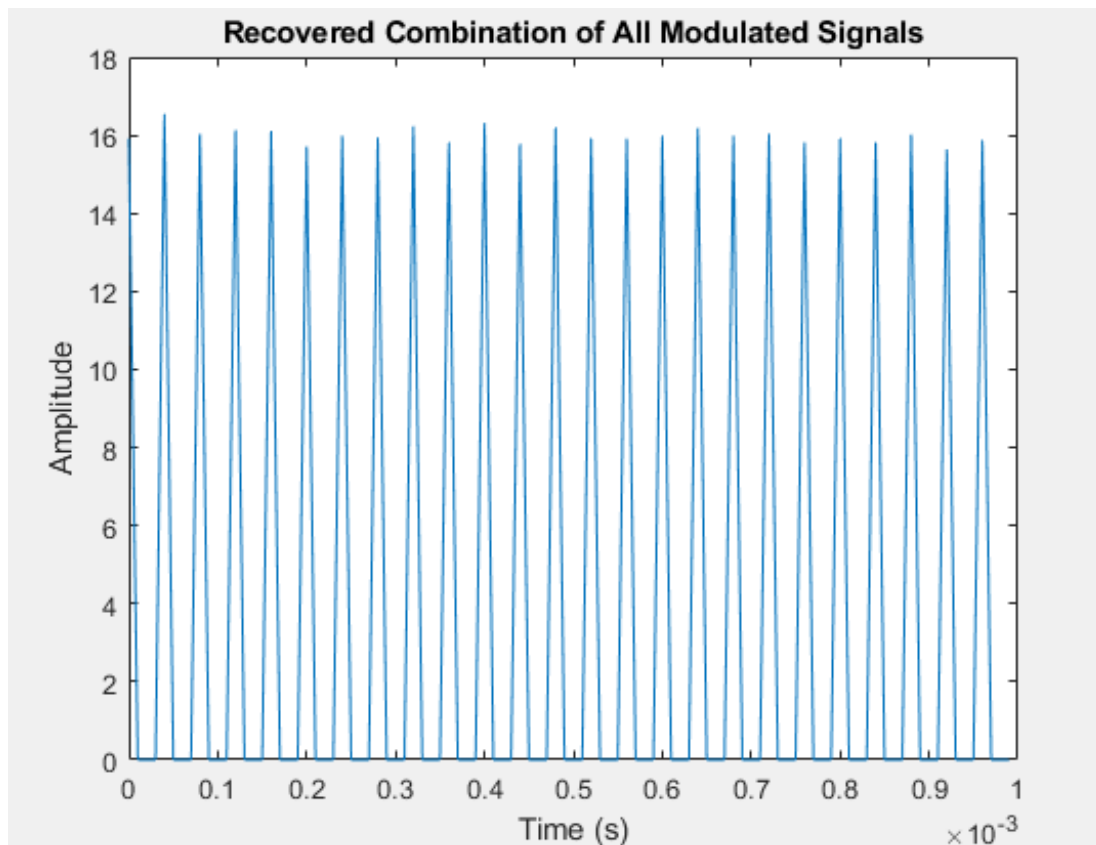
Slika 3.21: Graf obnovljenih moduliranih signala [izrada autora]
