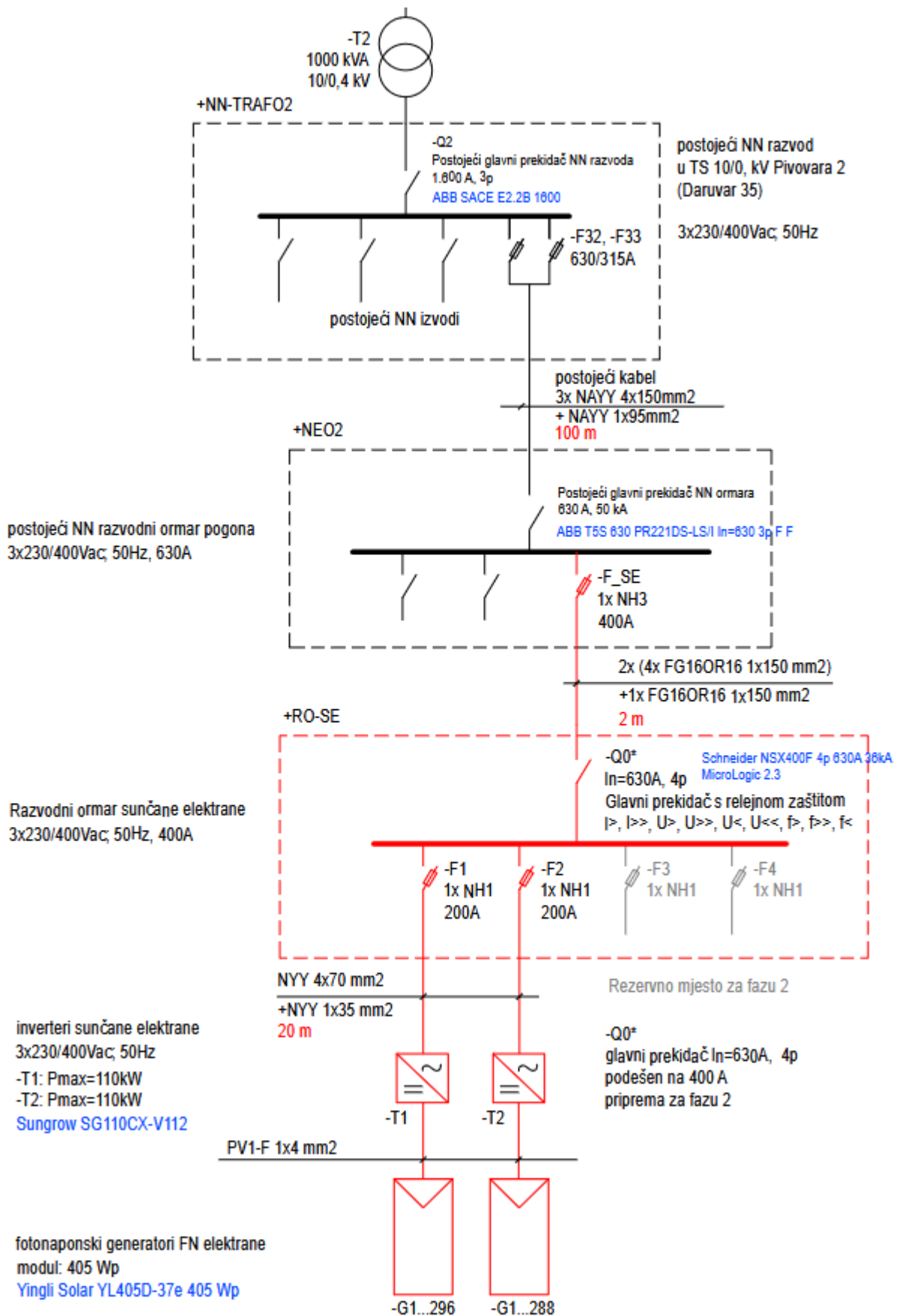
Slika 5.2. Jednopolna shema sunčane elektrane [14].
