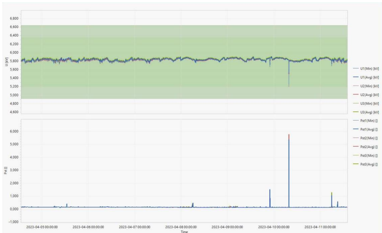
Slika 5.7. 10-minutne vrijednosti kratkotrajnog naponskog treperenja Pst (donji dijagram) te minimalnih 10 minutnih vrijednosti napona (gornji dijagram) u mjernom tjednu [14].
