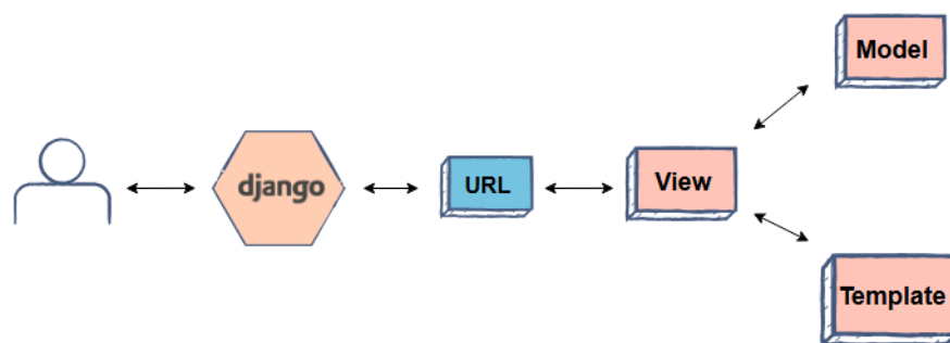
Slika 3.2. Prikaz toka podataka unutar MVT Django arhitekture [17]
