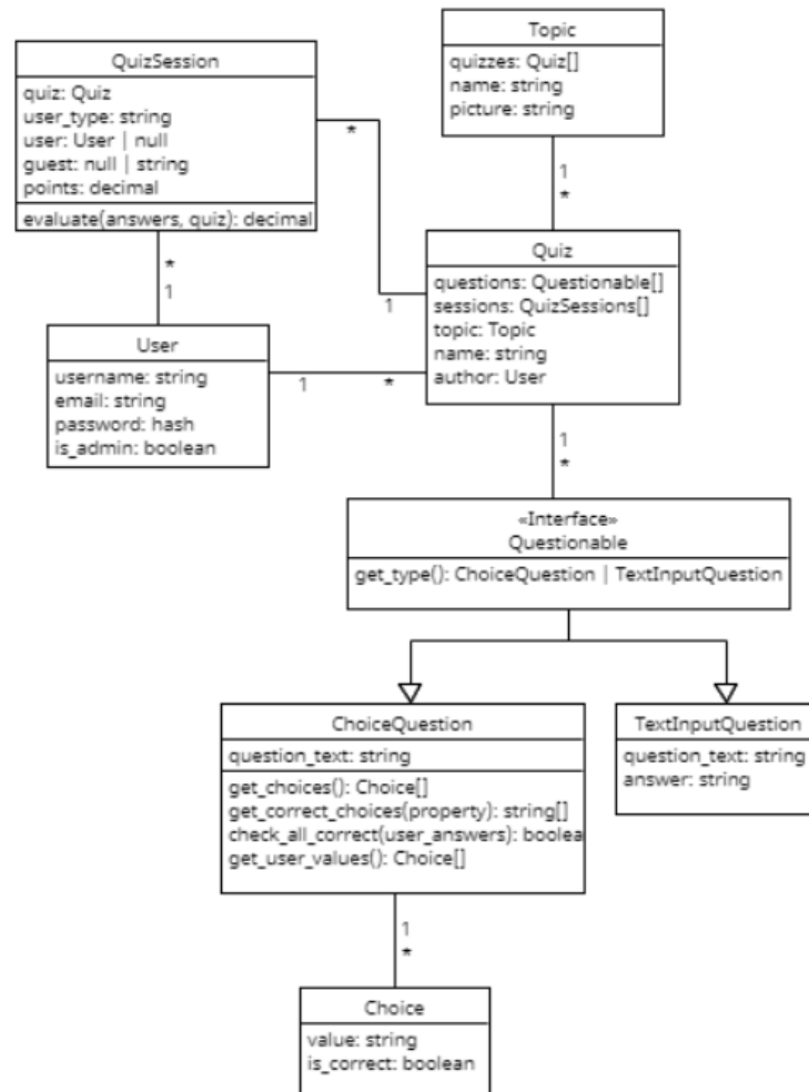
Slika 4.5. Prikaz dijagrama klasa
