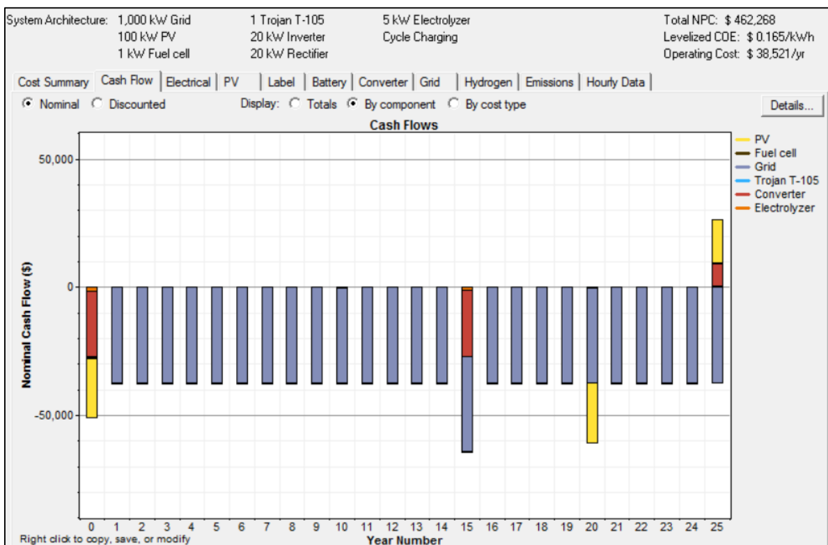
Sl. 5.16. Tijek novca kroz 25 godina
