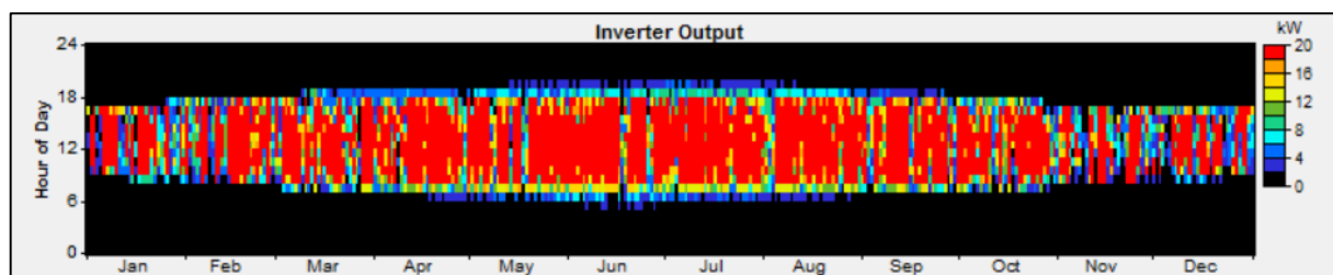
Sl. 5.27. Prikaz rada pretvarača kroz godinu
