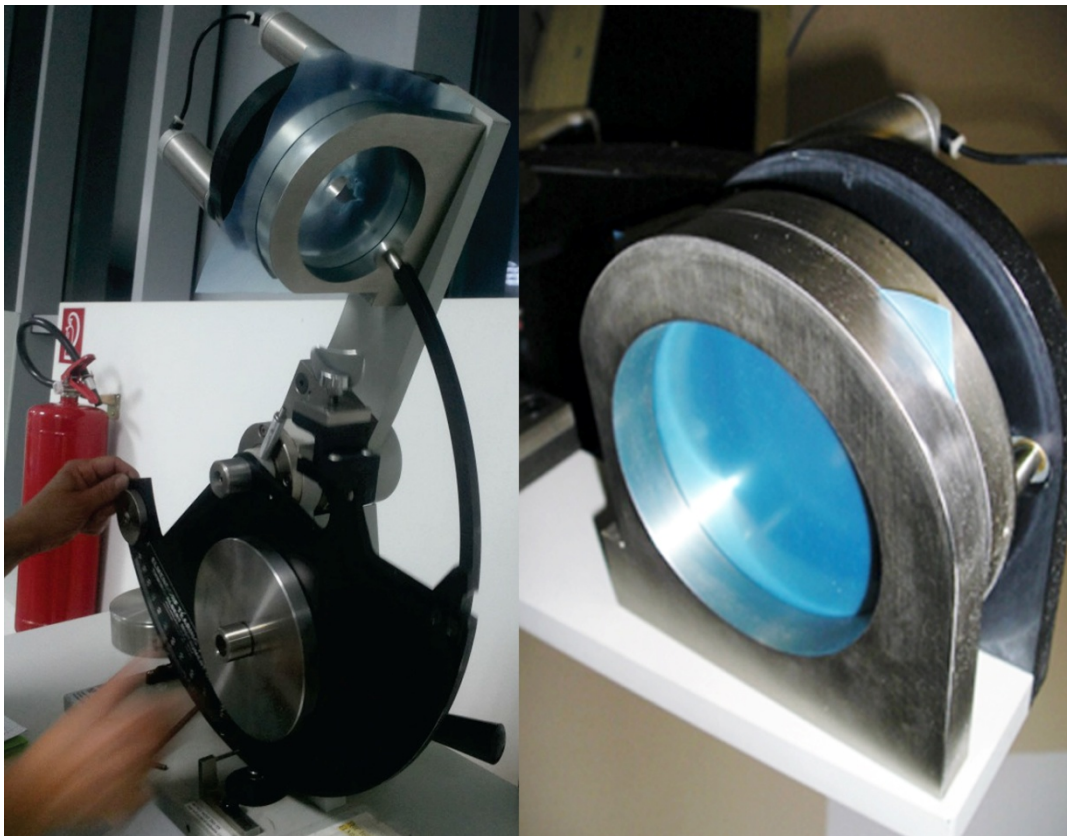
Slika 3.5.3.1. Test probijanja VpCI – 126 folije, [29].
