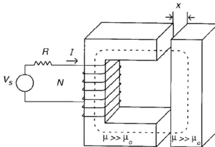
Slika 2.31. Složeni magnetski krug s dva zračna raspورا
