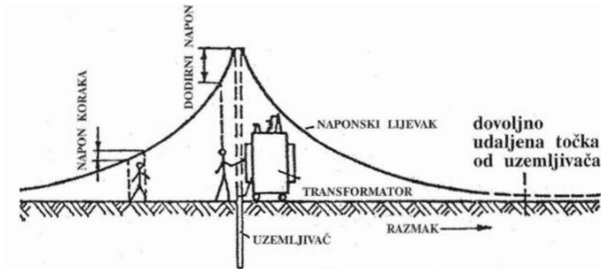
Slika 2.1) Razdioba potencija oko uzemljivača [2]
