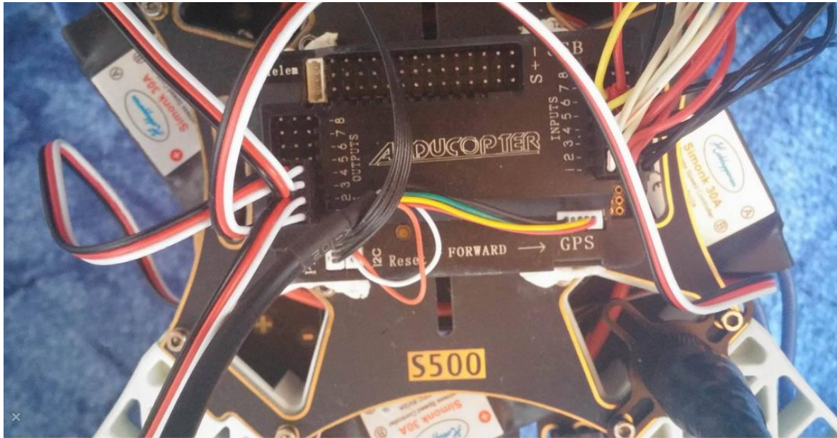
Slika 6.2. Kontroler arducopter
