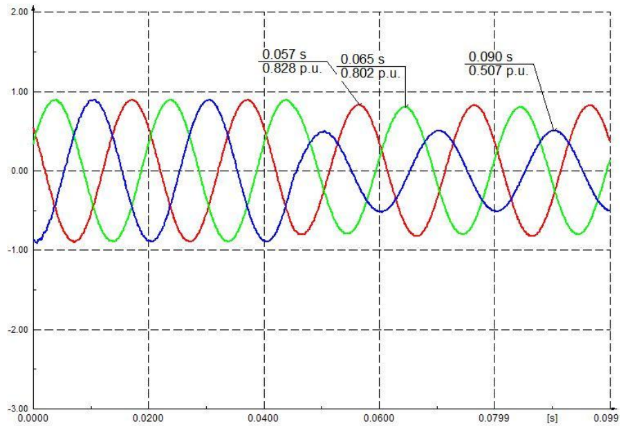
Sl. 3.37. Valni oblici napona pojedinih faza na sekundaru 20/0.4 kV za jednofazni kratki spoj
