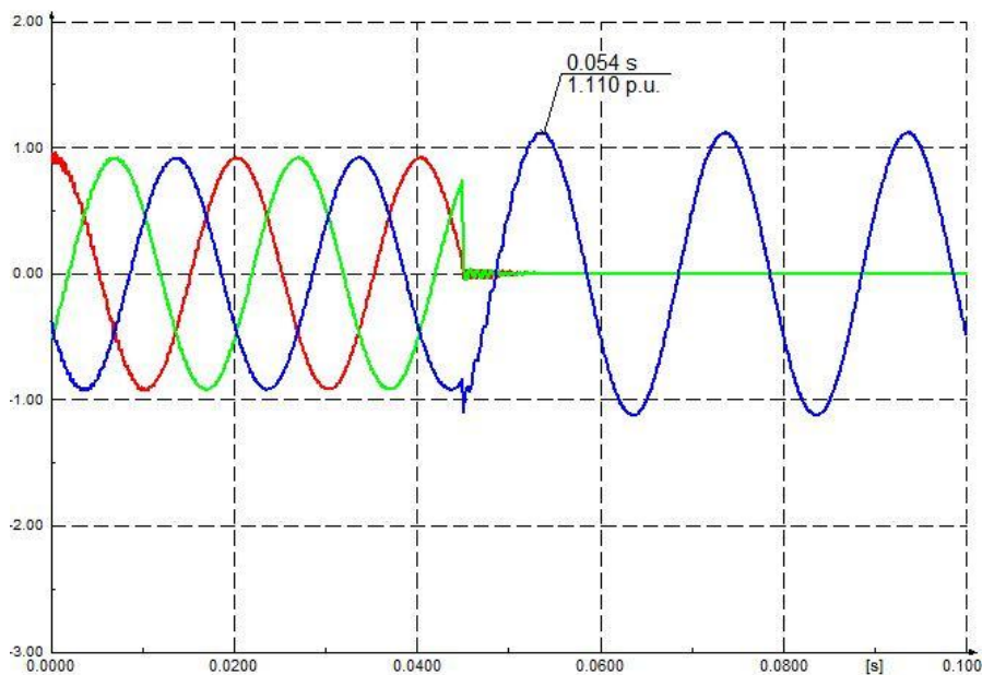
Sl. 3.13. Valni oblici napona pojedinih faza na primaru za dvofazni kratki spoj uz dodir sa zemljom
