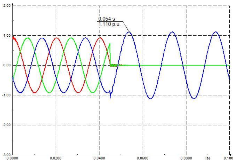
Sl. 3.19. Valni oblici napona pojedinih faza na primaru za dvofazni kratki spoj uz dodir sa zemljom
