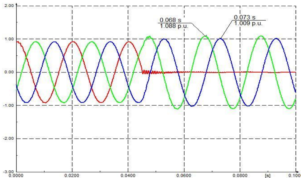
Sl. 3.4. Valni oblici napona pojedinih faza na sekundarnoj strani za jednofazni kratki spoj
