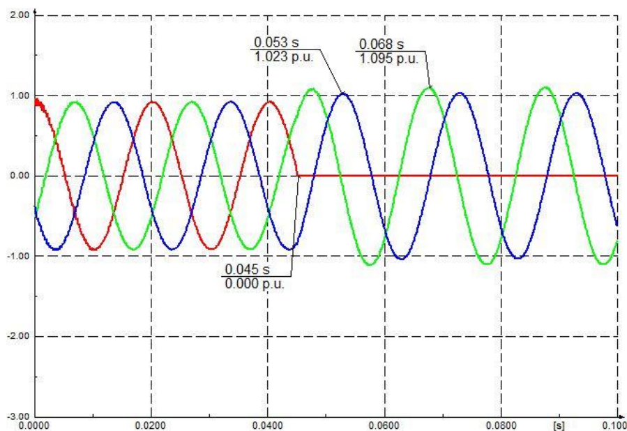
Sl. 3.17. Valni oblici napona pojedinih faza na primaru za jednofazni kratki spoj
