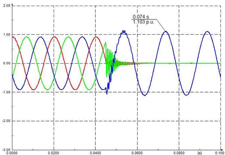
SI. 3.7. Valni oblici napona pojedinih faza na sekundaru za dvofazni kratki spoj uz dodir sa zemljom
