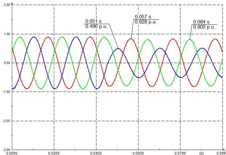
Sl. 3.30. Valni oblici napona pojedinih faza na sekundaru 20/0.4 kV za jednofazni kratki spoj
