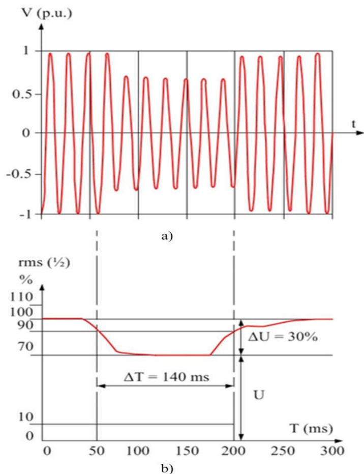
Sl. 2.10. Primjer naposnkog propada: a) vremenska domena, b) efektivna vrijednost[9]
