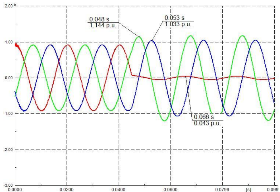
Sl. 3.26. Valni oblici napona pojedinih faza na primaru 35/20 kV za jednofazni kratki spoj
