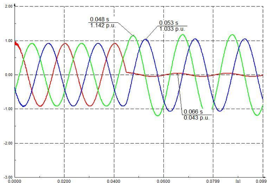
Sl. 3.33 Valni oblici napona pojedinih faza na primaru 35/20 kV za jednofazni kratki spoj
