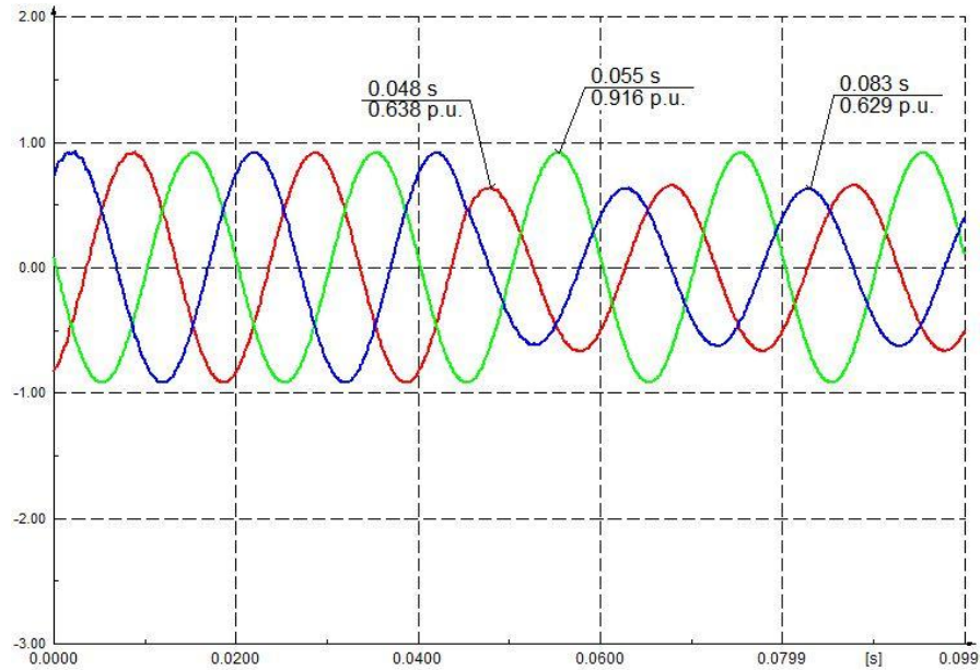
SI 3.34. Valni oblici napona pojedinih faza na sekundaru 35/20 kV za jednofazni kratki spoj
