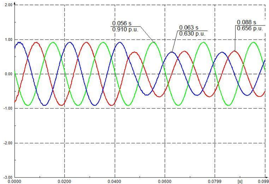
SI. 3.35. Valni oblici napona pojedinih faza na primaru 20/0.4 kV za jednofazni kratki spoj
