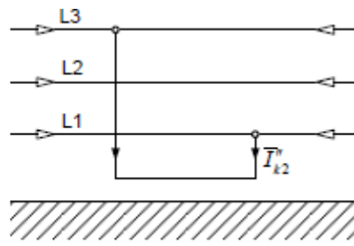
SI. 2.4. Dvofazni kratki spoj[2]
