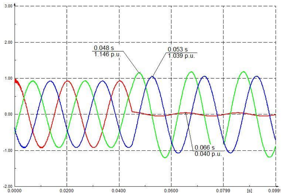
Sl. 3.25. Valni oblici napona pojedinih faza na sekundaru 110/35 kV za jednozadni kratki spoj
