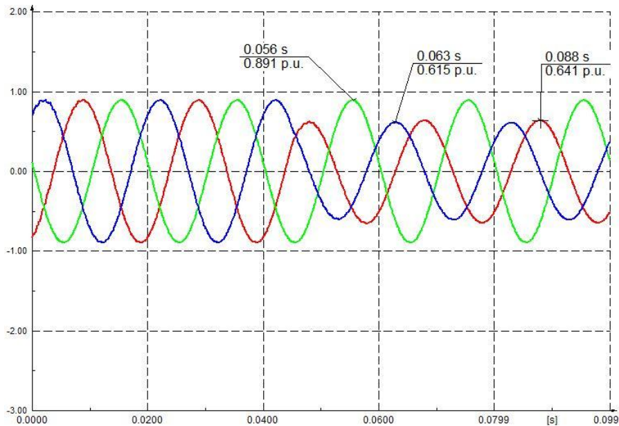
Sl. 3.29. Valni oblici napona pojedinih faza na sekundaru 20/0.4 kV za jednofazni kratki spoj
