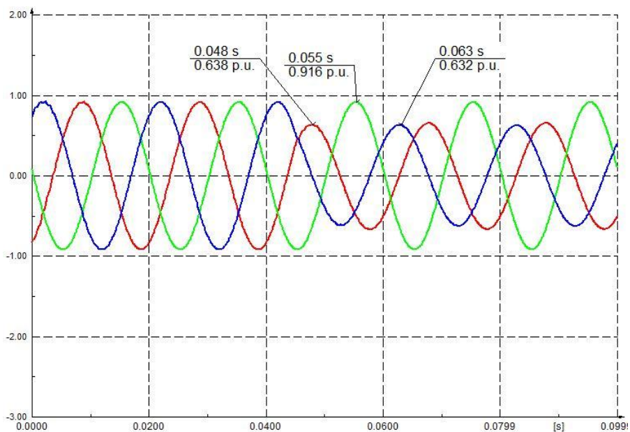
Sl. 3.27. Valni oblici napona pojedinih faza na sekundaru 35/20 kV za jednofazni kratki spoj
