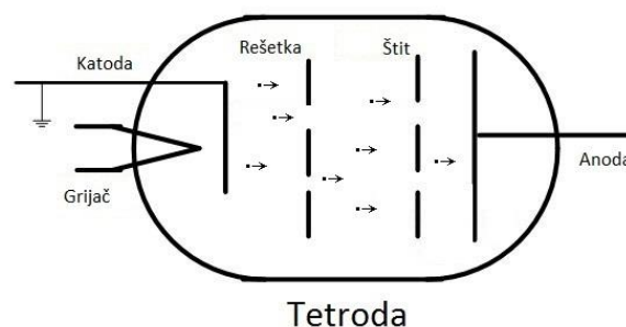
Slika: 2.4 Tetroda [4]
