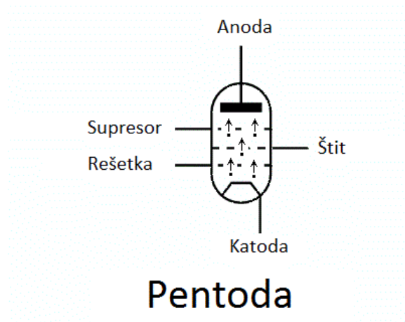
Slika 2.5: Pentoda [5]
