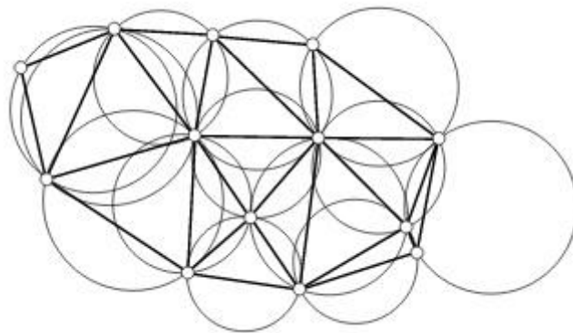
Slika 3.1. Svaki trokut u Delaunayevnoj triangulaciji ima praznu opisanu kružnicu (Slika preuzeta iz [6])
