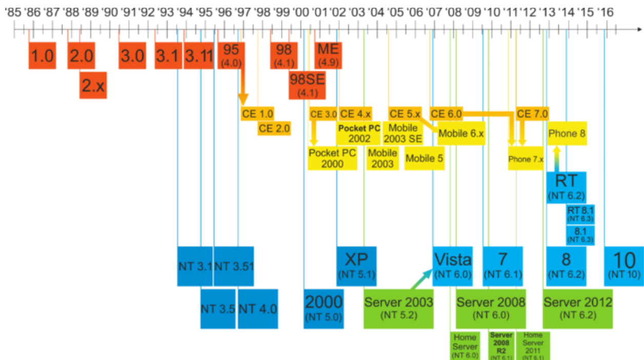
Slika 2.2: Vremenska lenta Microsoft Windows operativnih susava [6]
