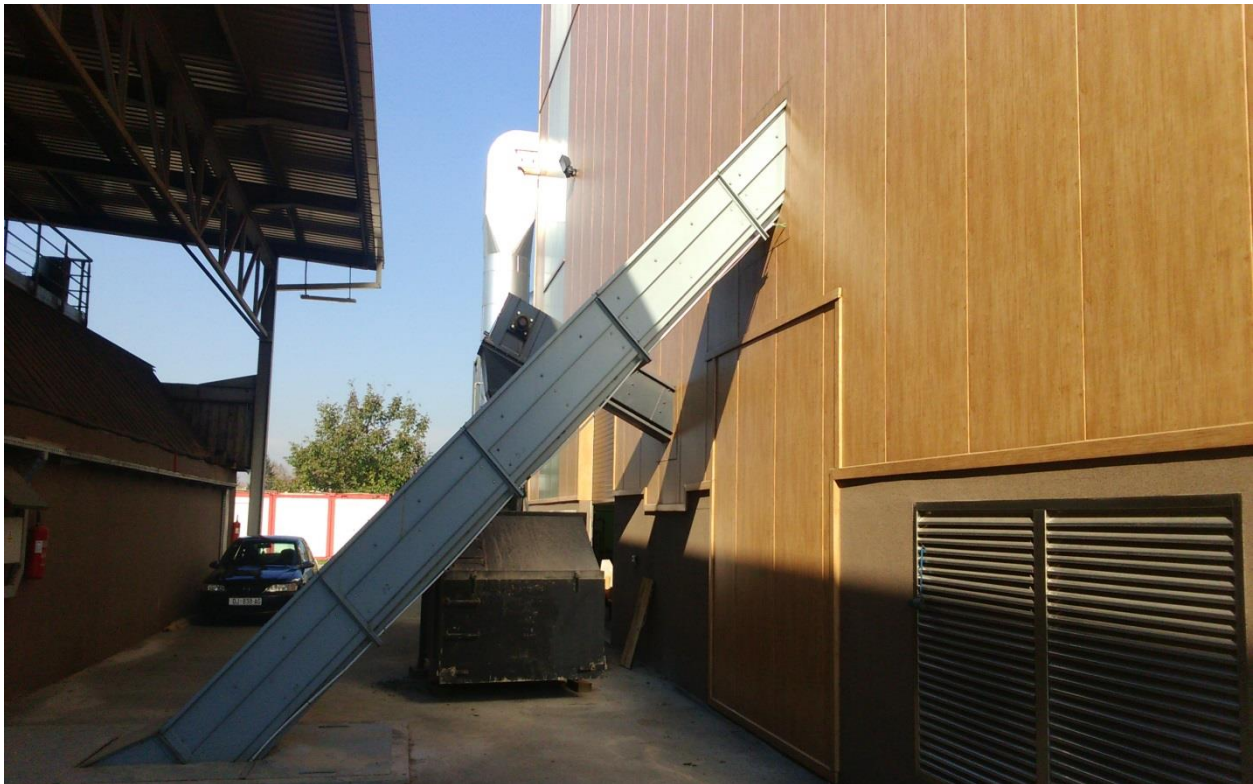
Slika 5.3. Lančani transporter
