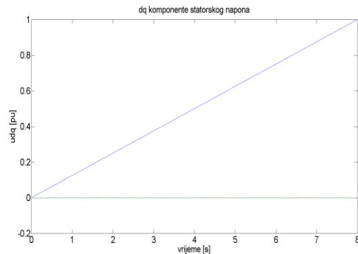
Sl. 4.14. Statorski napon u dq sustavu
