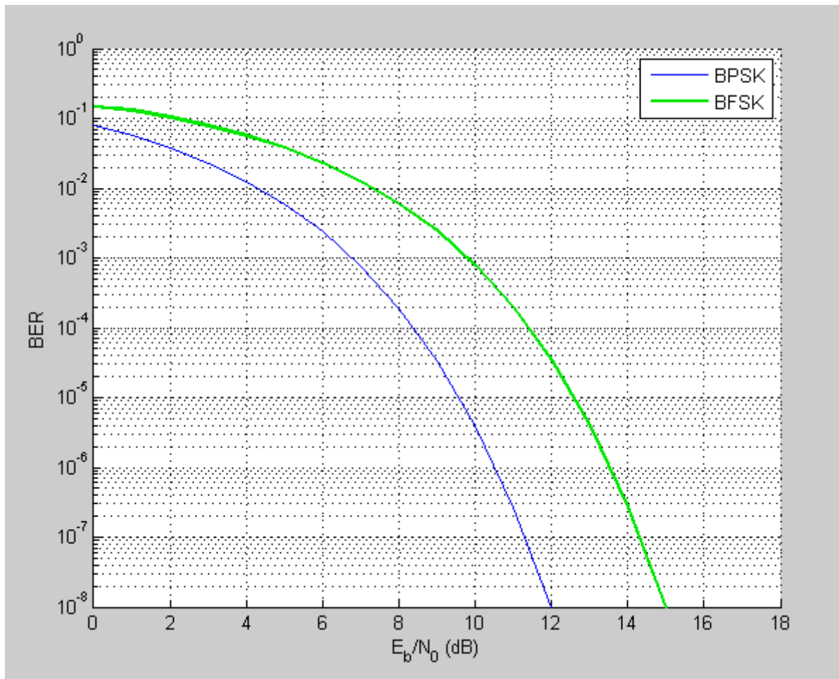
Sl.3.4. Bertool simulacija BPSK i BFSK
