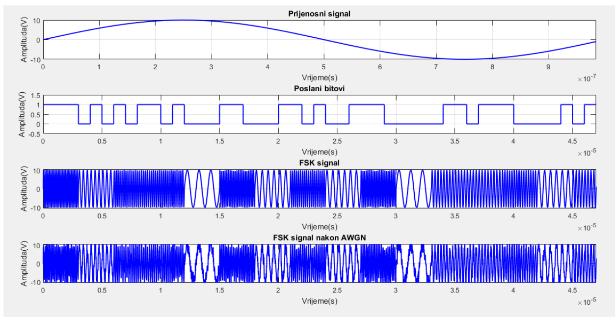
S1.3.3. FSK modulacija
