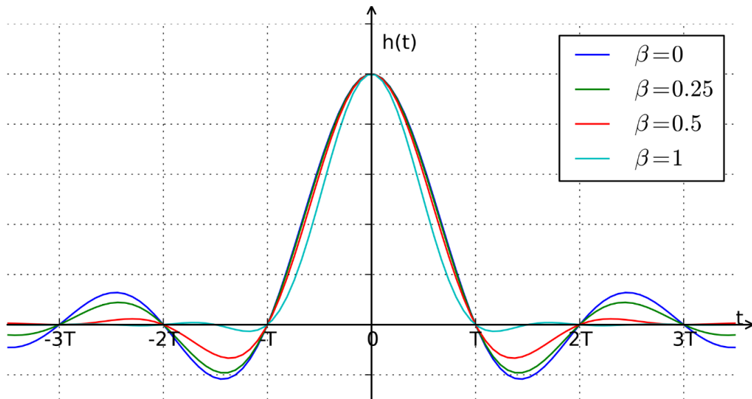
Sl.2.6. Impulsni odziv filtra s kosinusno zaobljenom karakteristikom [8]
