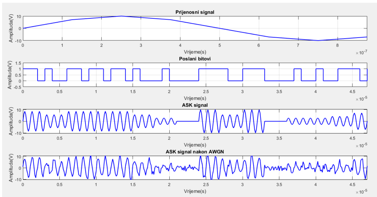
S1.3.1. ASK modulacija
