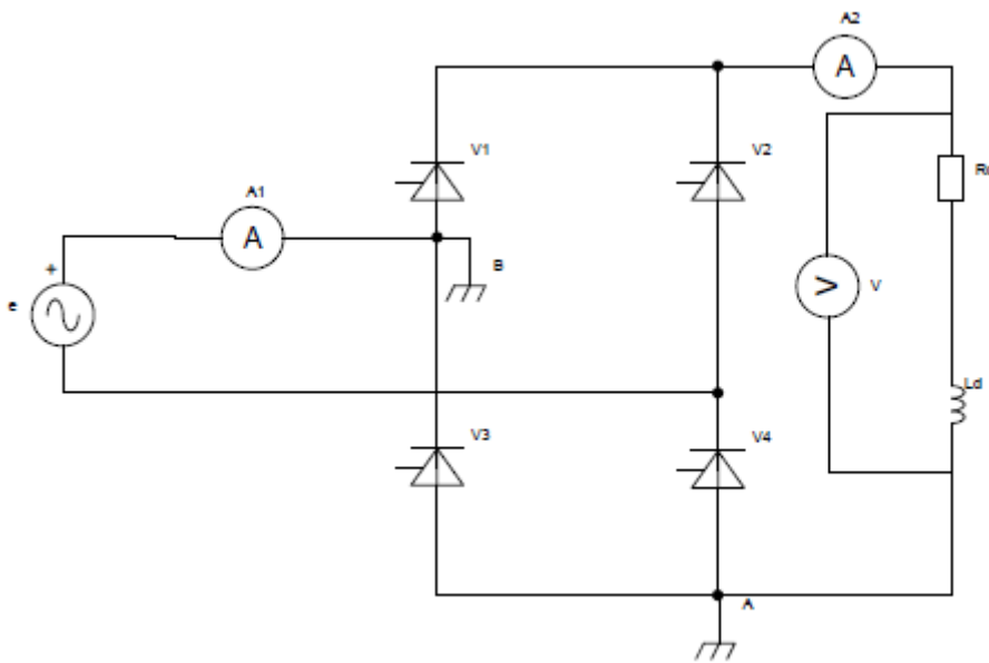
Slika 4.1 Shema mjerenja
