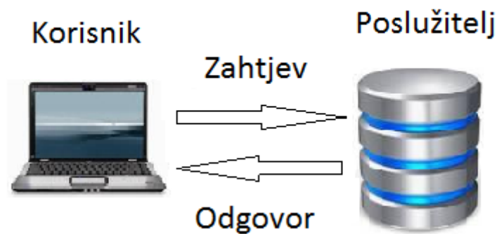
Slika 4.2.1. Dvoslojna arhitektura
