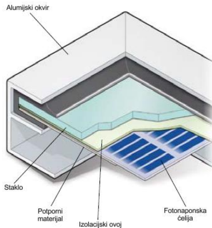
Slika 3.8. Presjek standardnog fotonaponskog modula. [8]
