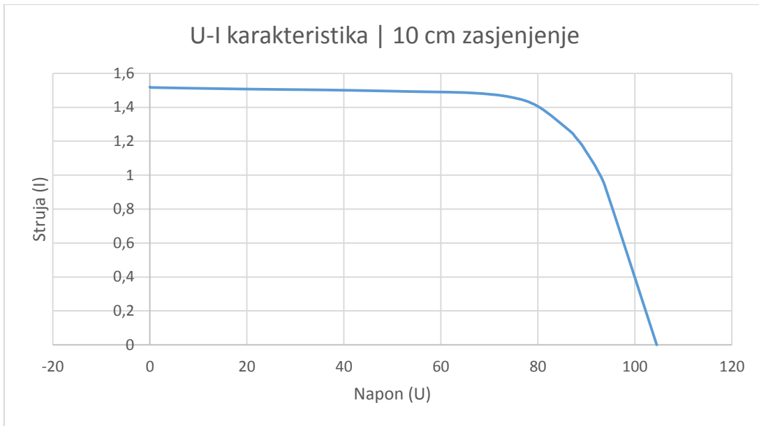
Slika 5.15. U-I karakteristika pri zasjenjenju fotonaponskog modula SOLAR FRONTIER SF-150 od 10 cm.
