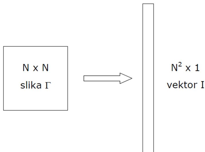
Sl. 7.1.1 Prikaz slike u jednoj dimenziji (Izvor : http://stephenpaulraj.com/face-detectionrecognition-eigenfaces/ )
