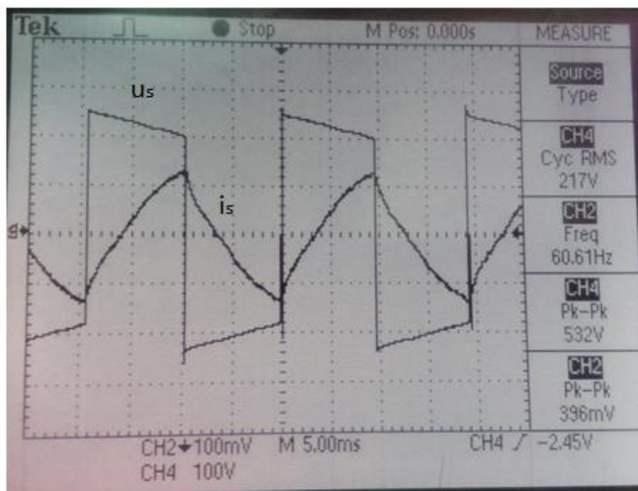
Slika 5.13. Valni oblik napona u_s i struje i_s .
