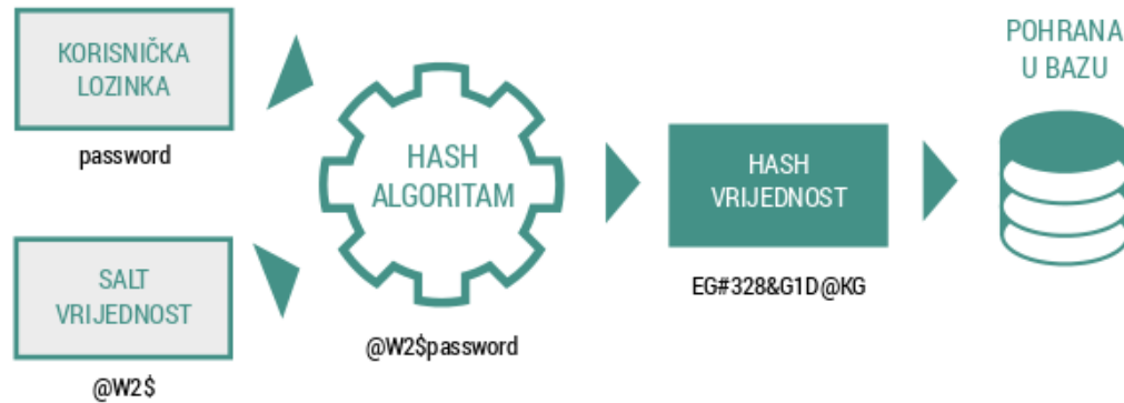
Sl. 4.1. Način rada hash funkcije
