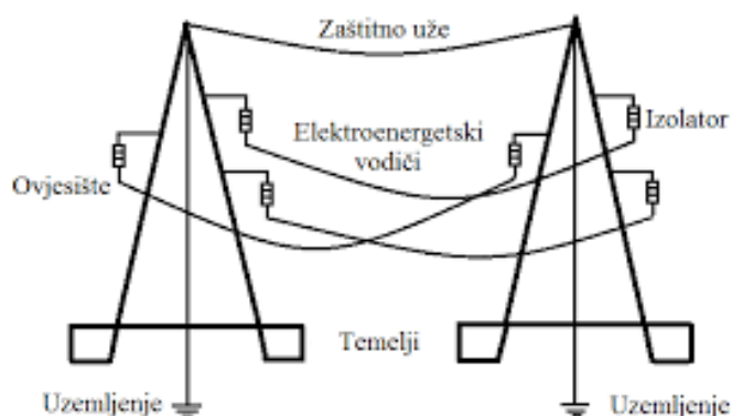
Slika 2.1. Nadzemni vodovi
