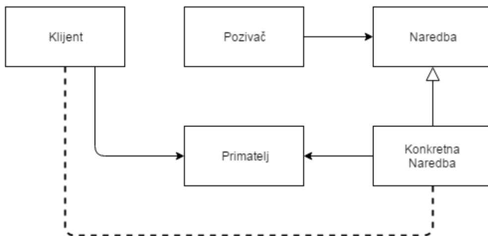
Slika 2.13. Struktura Naredbe
