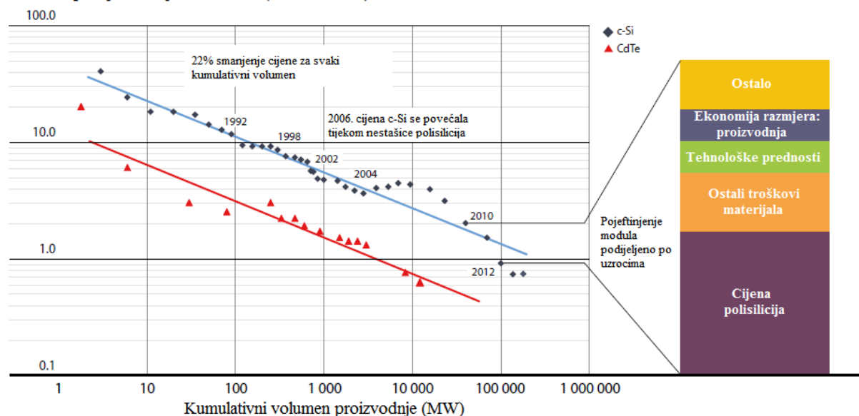
Slika 3.11. Prosječna globalna cijena FN modula kroz povijest za c-Si i CdTe module [12]
