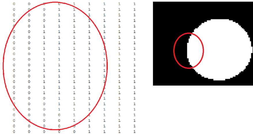
Slika 2.2 Binarna slika
