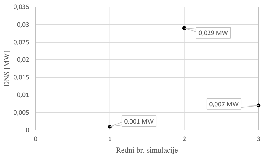
Slika 4.17 Zbirni grafički prikaz srednjih vrijednosti konvergencija varijable DNS između simulacija
