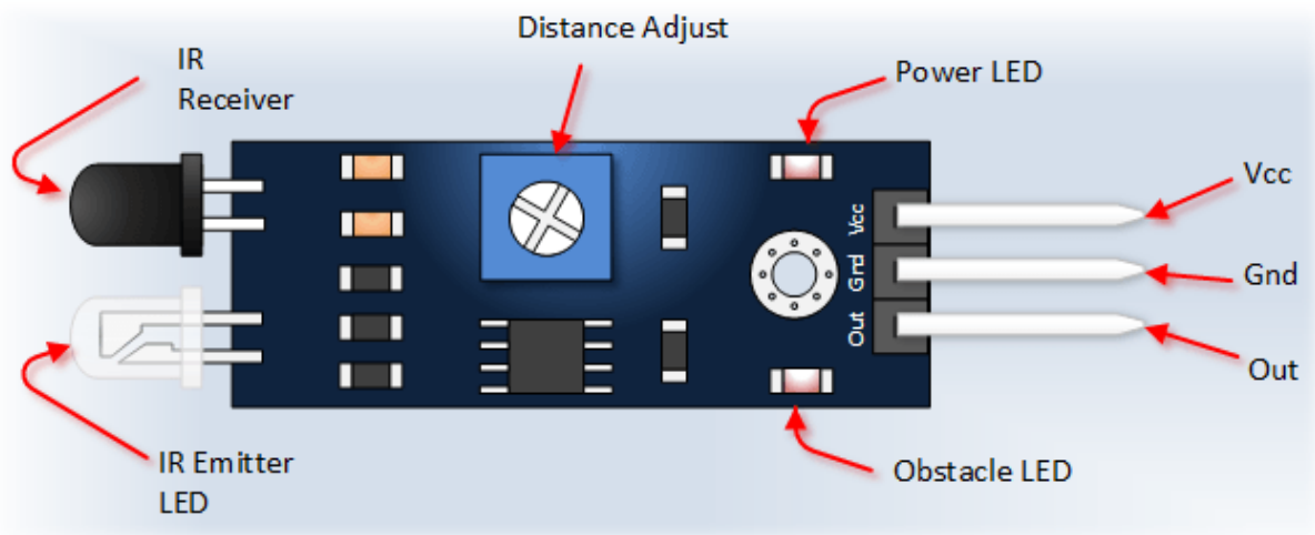
Slika 3.3. Infracrveni senzor.
