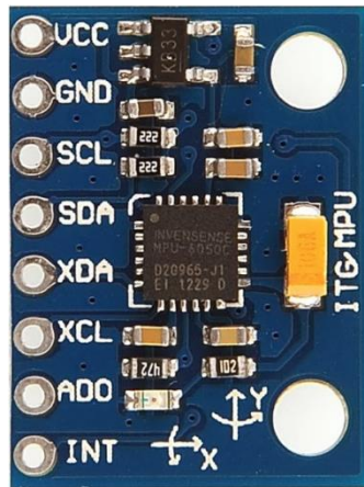
Sl. 4.6. Akcelerometar MPU-6050[19]
