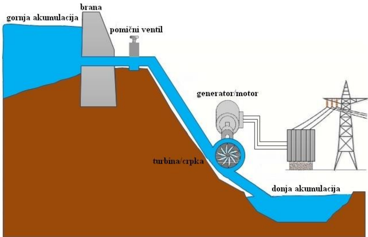
Slika 2.4. Reverzibilna hidroelektrana [22]
