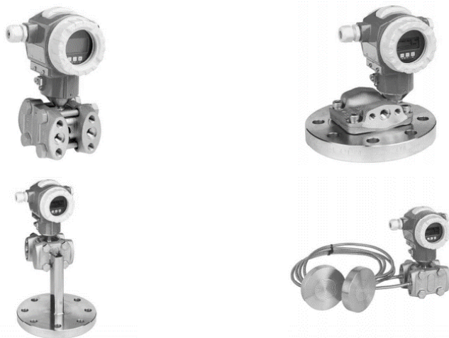
Sl.3.10. Mjerenje razine otvorenog spremnika Sl.3.11. Izvedbe hidrostatskih mjerila razine
