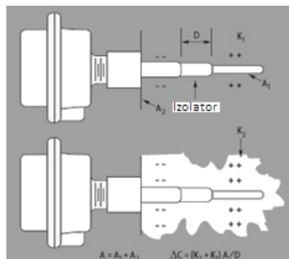
SI.3.48. Horizontalno smješteno kapacitivno osjetilo razine
