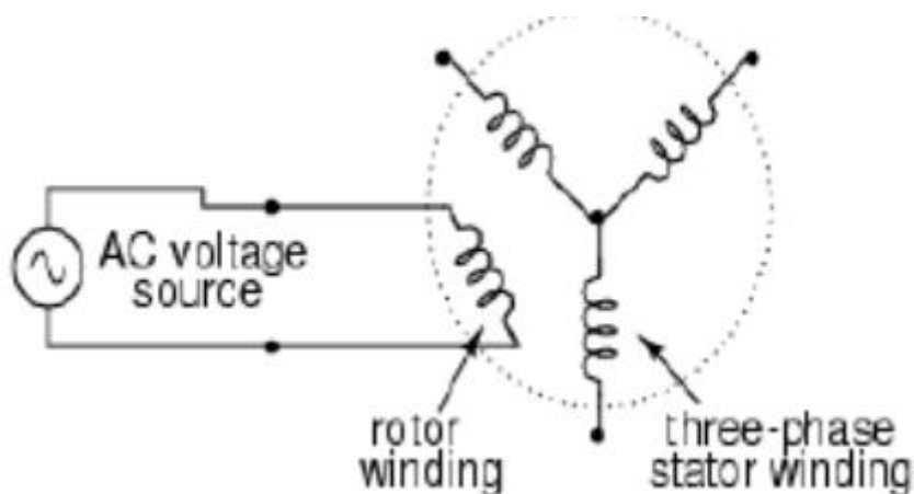
Sl. 2.8. Shematski prikaz Synchra [5].
