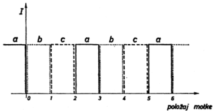
Sl. 2.4. Redoslijed struja statora za pomicanje prema gore [12].
