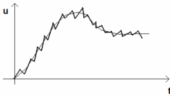
Sl. 3.5. Šum tahogeneratorsa[8].
