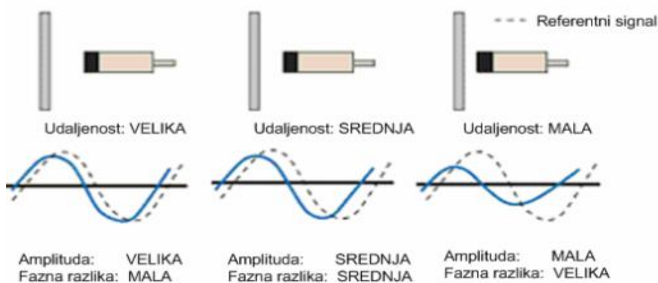
Sl. 2.12. Utjecaj udaljenosti na amplitudu i fazni pomak[6]
