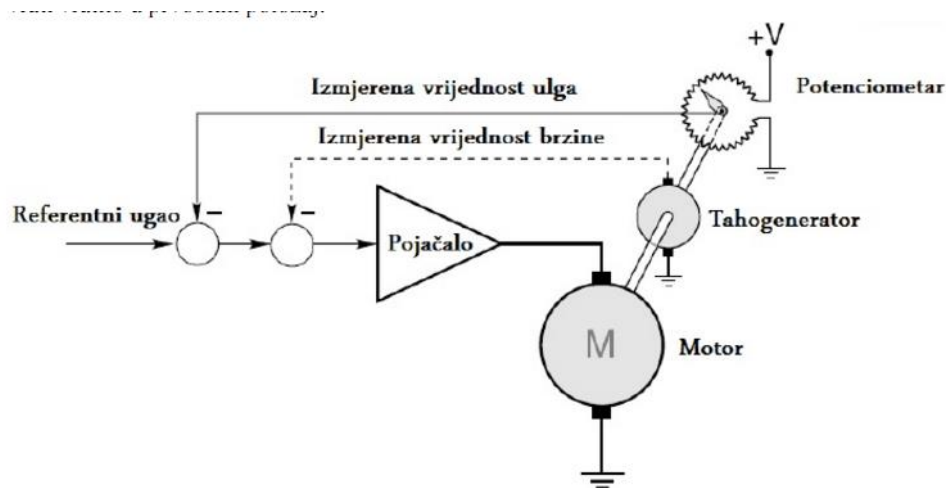
Sl. 4.4. Servomehanizam [12].
