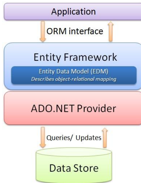
Sl. 3.3. Arhitektura Entity Framework-a [8]
