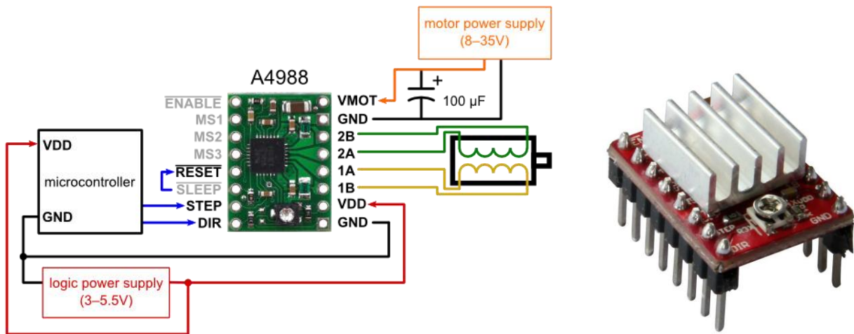
Slika 4.15. Driver koračnih motora A4988 [2]
