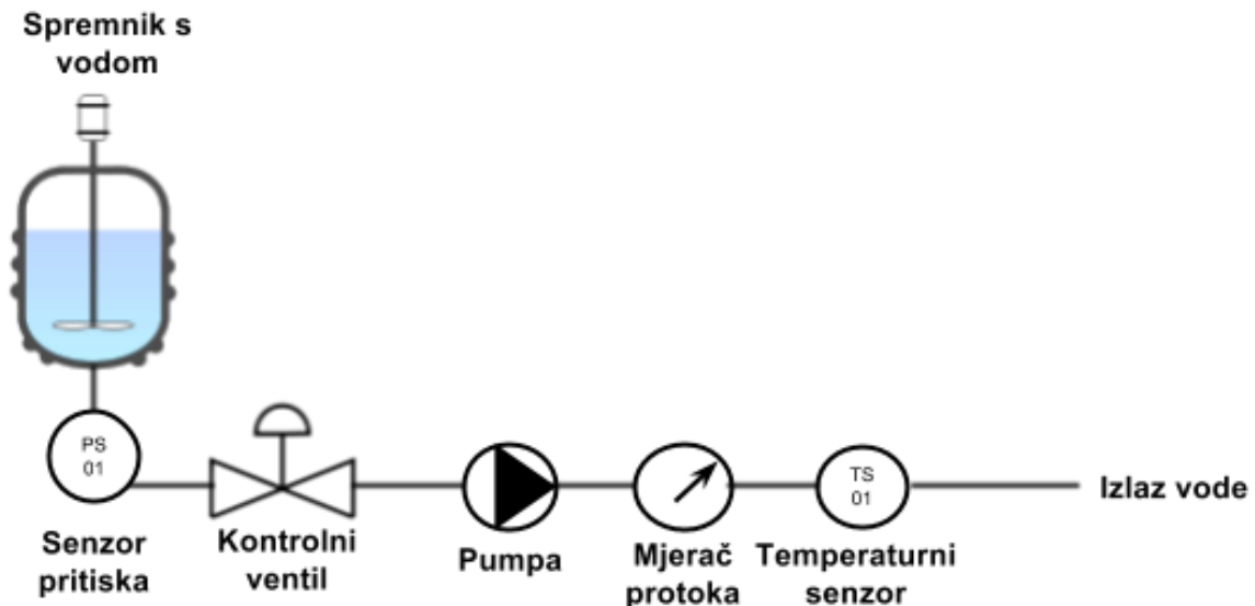
Slika 3.6: Shema spajanja mjernih i izvršnih članova u sustavu navodnjavanja.
