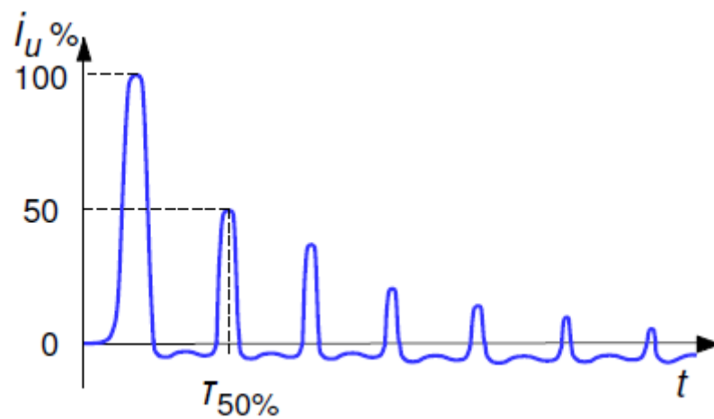
Slika 2.1. Struja uklapanja [2]
