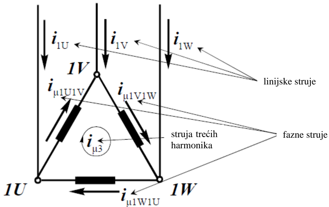
Slika 3.6. Struje magnetiziranja kod spoja transformatora u trokut [8]
