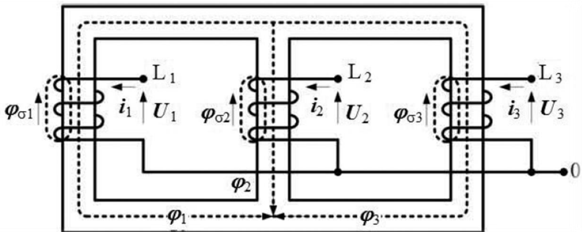
Slika 2.4. Pojednostavljena shema trofaznog transformatora u praznom hodu [6]
