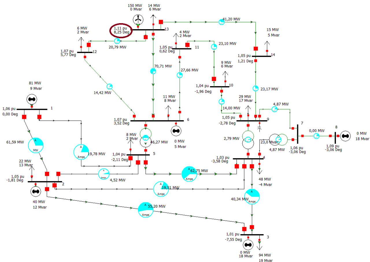
Sl. 6.18. Priključak vjetroelektrane na sabirnicu 13
