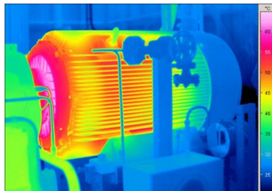
Slika 2.1. Primjer termovizijske snimke elektromotora.[3]
