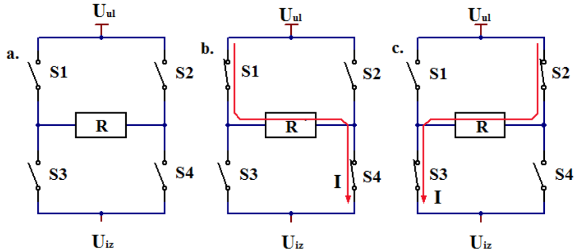
Slika 4.3. Prikaz H-mosta [11]
