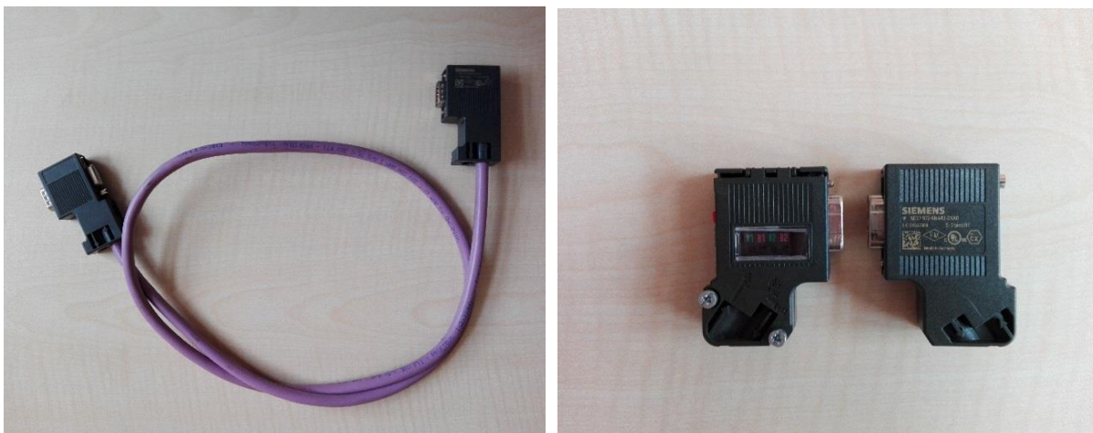
Slika 3.7. Oklopljeni dvožični vod (lijevo) i D-sub konektor (desno)
