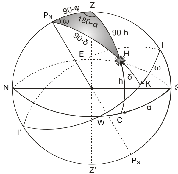
Slika 4.6. Nebeska sfera [14]
