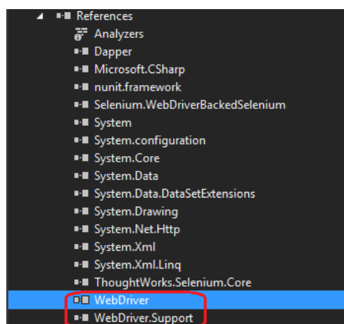
Slika 4.5 WebDriver DLL
